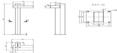
Рисунок 2. Общий вид светильника
